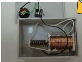
ソレノイドをつかえば、ドラムやベル、いろいろなものが叩けちゃう。
